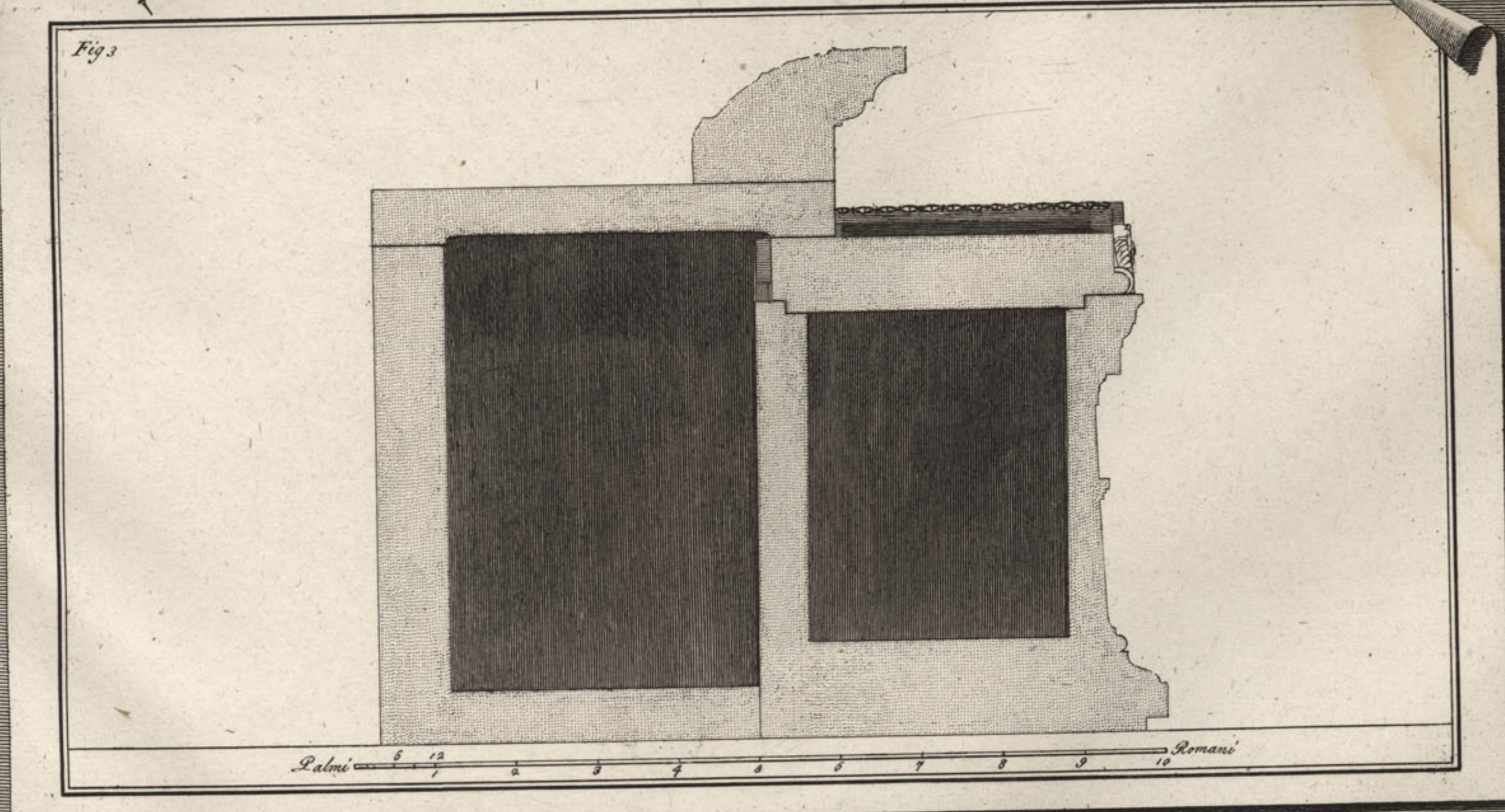
Prospetto esteriore del Monumento degli Scipioni collo spaccato de Sarcofagi di Scipione Barbato, e d'Aula Cornelia Cav. Giovanni Finazzi f.
