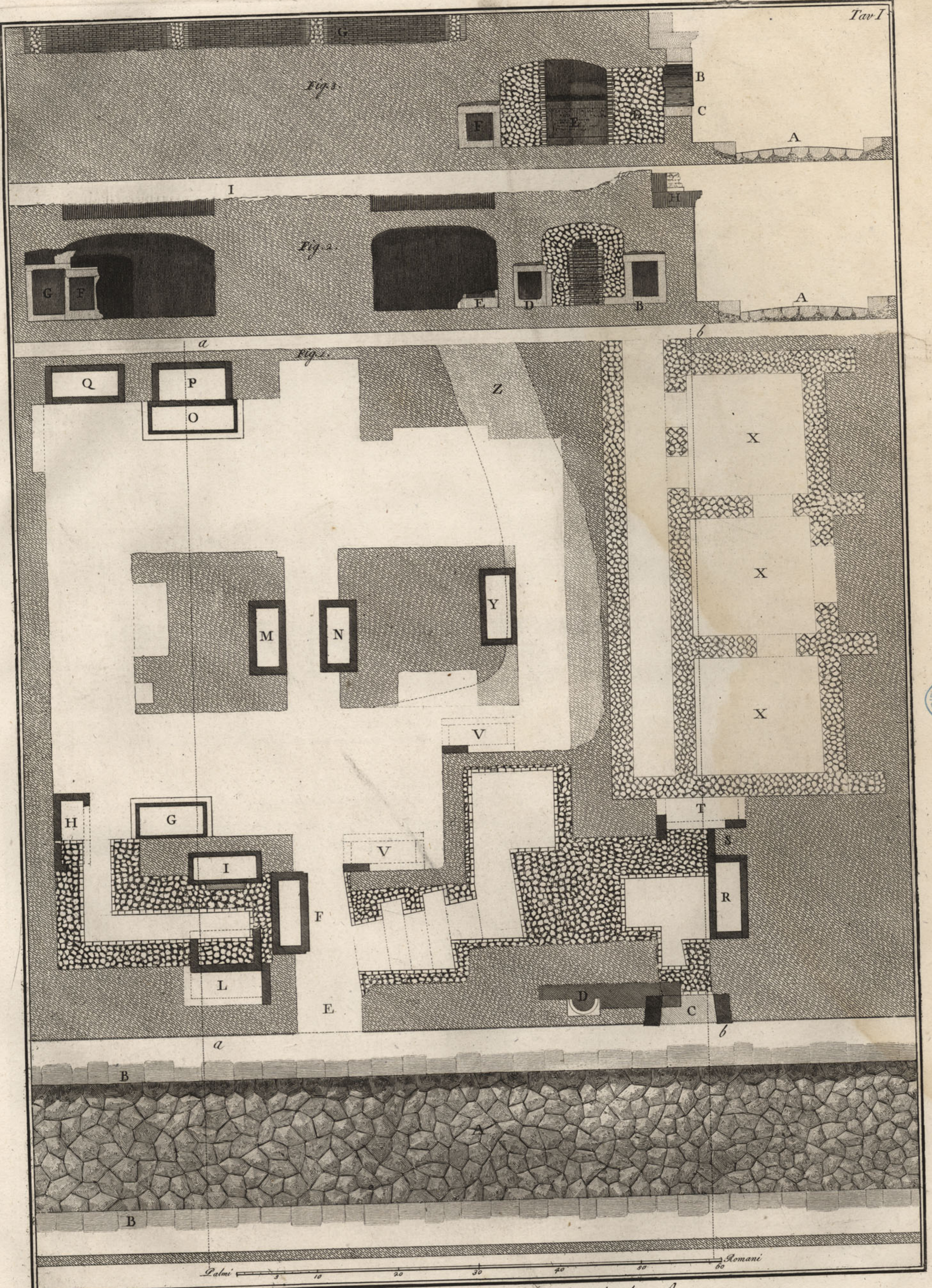
Pianta e spaccati dell' Stoa degli Scipioni
