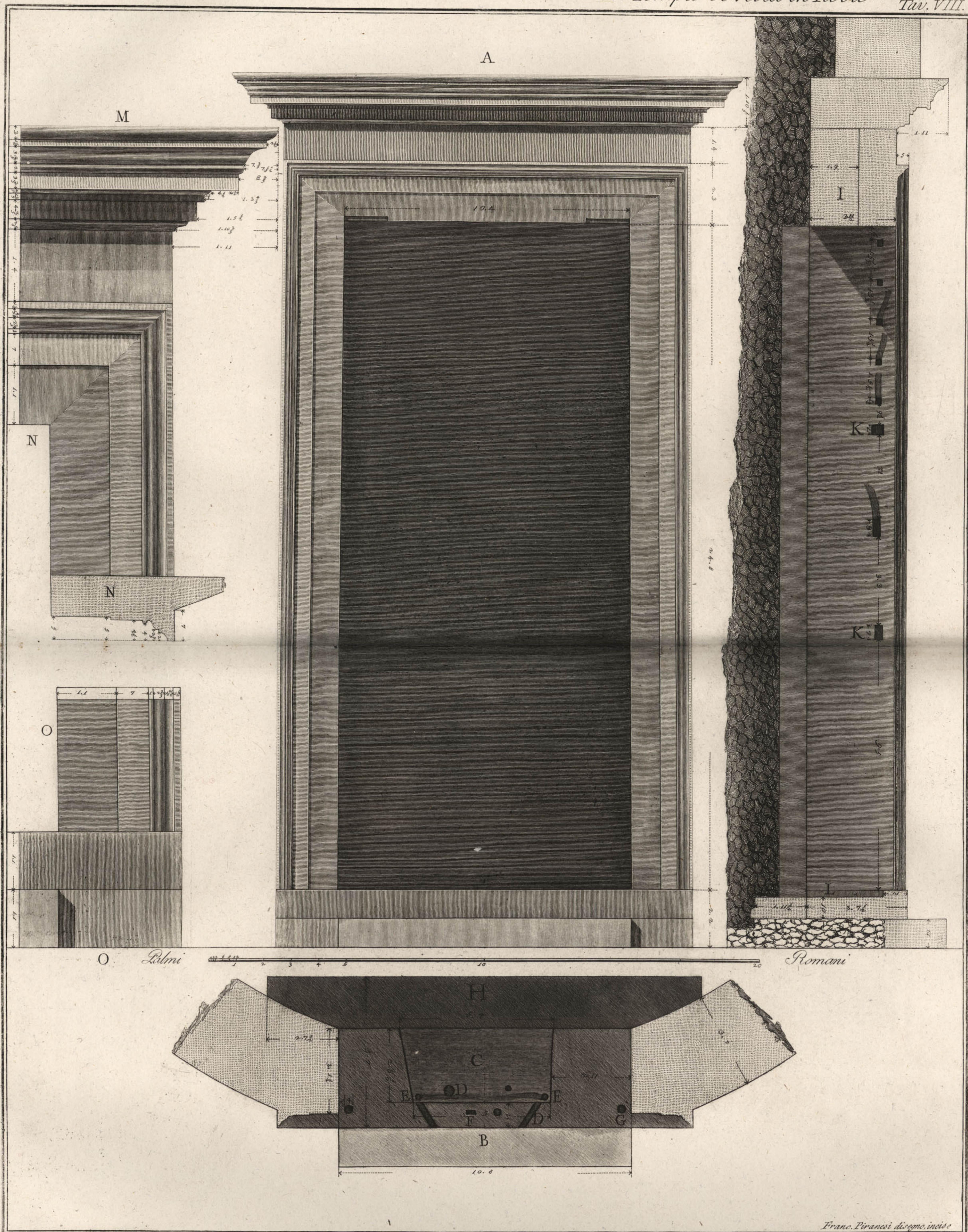
A Porta a campana già ornata con bustole di bronzo. B Pianta della medesima. C Incastro nel liminare o soglia, che riceveva una tavola di bronzo. Il medesimo stabilisce le larghezze delle valve, che si aprivano di dentro. D Canali, e fori, che fissavano i grappi della tavola suddetta. E Fori per ritenere i cardini. F Altri che incassavano il chiavistello per assicurare le valve contro il battente nel liminare. G Fori per fermare l'intavolamento del telaio della porta. H Parte del litistrato o Pavimento interno della Cella a livello dell'incastro C. I Profilo dello stipite, che indica i fori K, i quali tenevano l'intavolamento del telaio della porta ora slabrati dallo sforzo di scuoterla allor quando fu tolta. L Incastro nella soglia, che riteneva la tavola di bronzo suddetta. M Cornice o fregio di scala maggiore. N Modinatura dell'architrave, e sua pianta. O Stipite coll'indicazione dell' due gradi.
