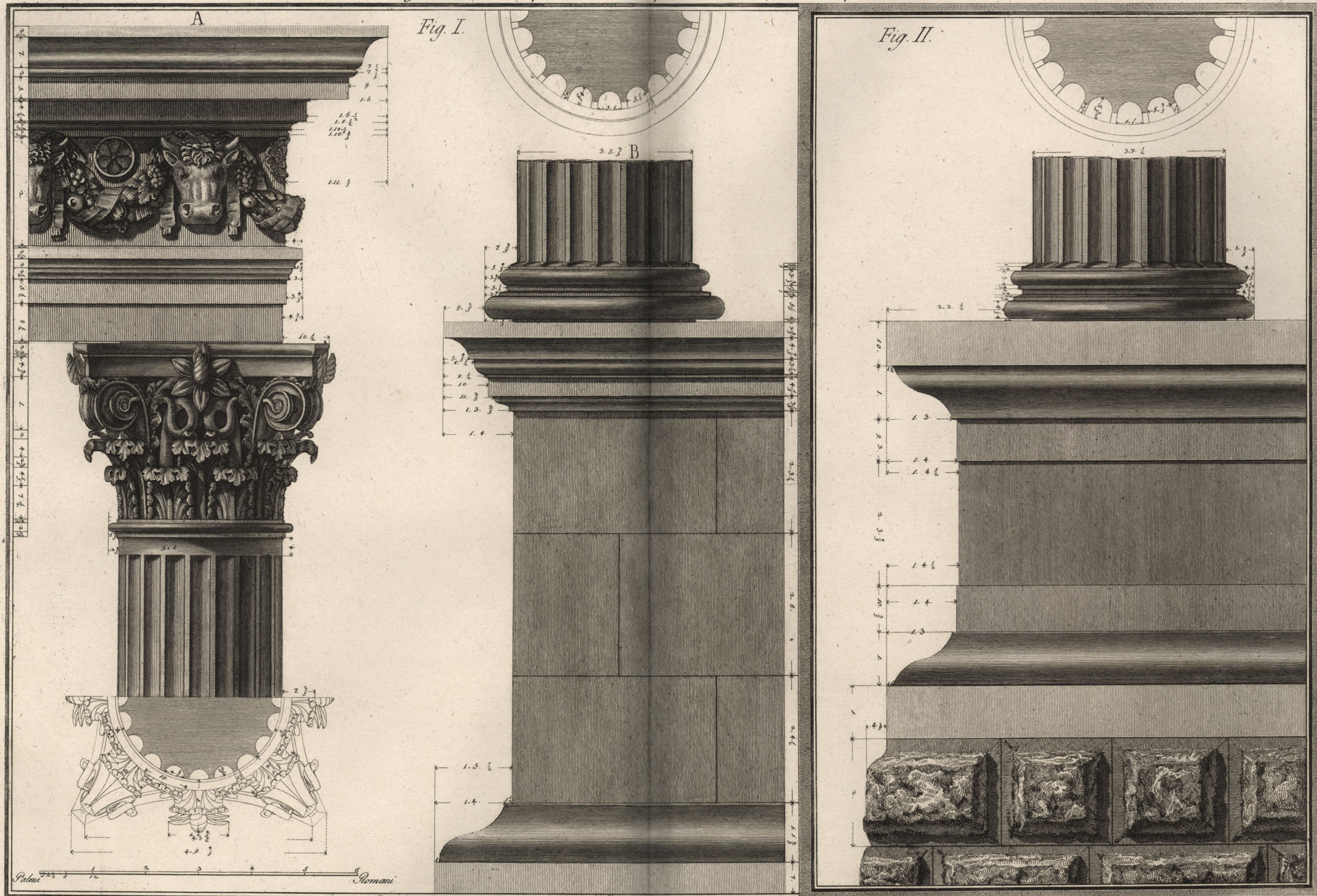
Figura I. A. Modinature della Cornice, fregio, Architrave, Capitello, e sommoscapo della Colonna, e sua pianta del Tempio di Vesta in Tivoli. B. Modinature del Basamento, Cimasa, base, e imoscapo della Colonna, e pianta.
