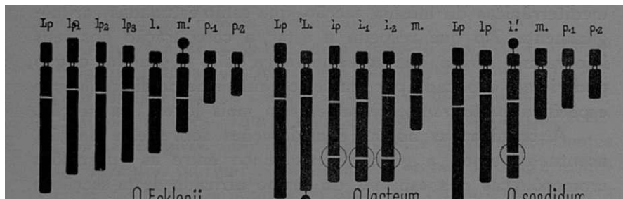
Fig. 9 — Representação esquemática das guarnições cromosómicas de O. Ecklonii Schlecht., O. lacteum Jacq. e O. sordidum Baker. As dimensões dos cromosomas são as médias de 10 placas metafásicas de cada uma das espécies. \times 3600 .
