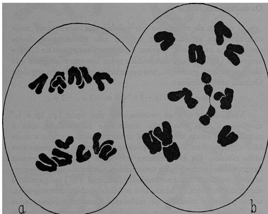
Fig. 3 — O. lacteum Jacq. Anafase I. Alcool acético-carmim acético. X 1800.
