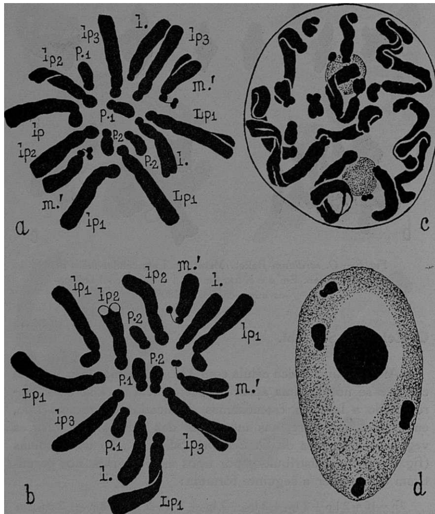
Fig. 7 — O. Ecklonii Schelecht. a, b , Metafases em células dos vértices vegetativos das raízes mostrando 2n = 16 ; c , Profase, notando-se os cromosomas m.' ligados aos nucléolos; d , Núcleo em intercinese, mostrando 4 cromocentros correspondentes aos 4 heterocromatinosomas. Navachine-violete de genciana. X 3600.
