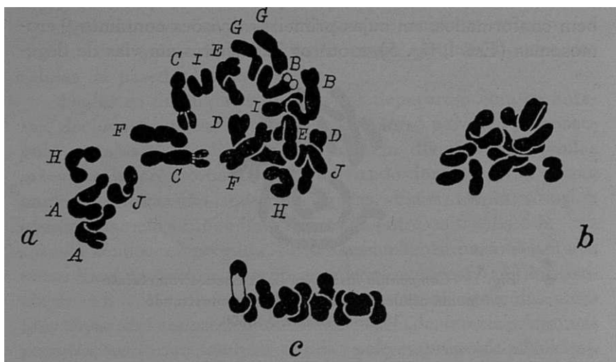
Fig. 2 — Campanula transtagana R. Fernandes. a , Metafase em uma célula da parede da antera, mostrando 20 cromosomas cujos pares são indicados pelas letras A-J. b , Metafase num grão de pólen. c , Metafase I com 10 bivalentes. \times 3200 .
