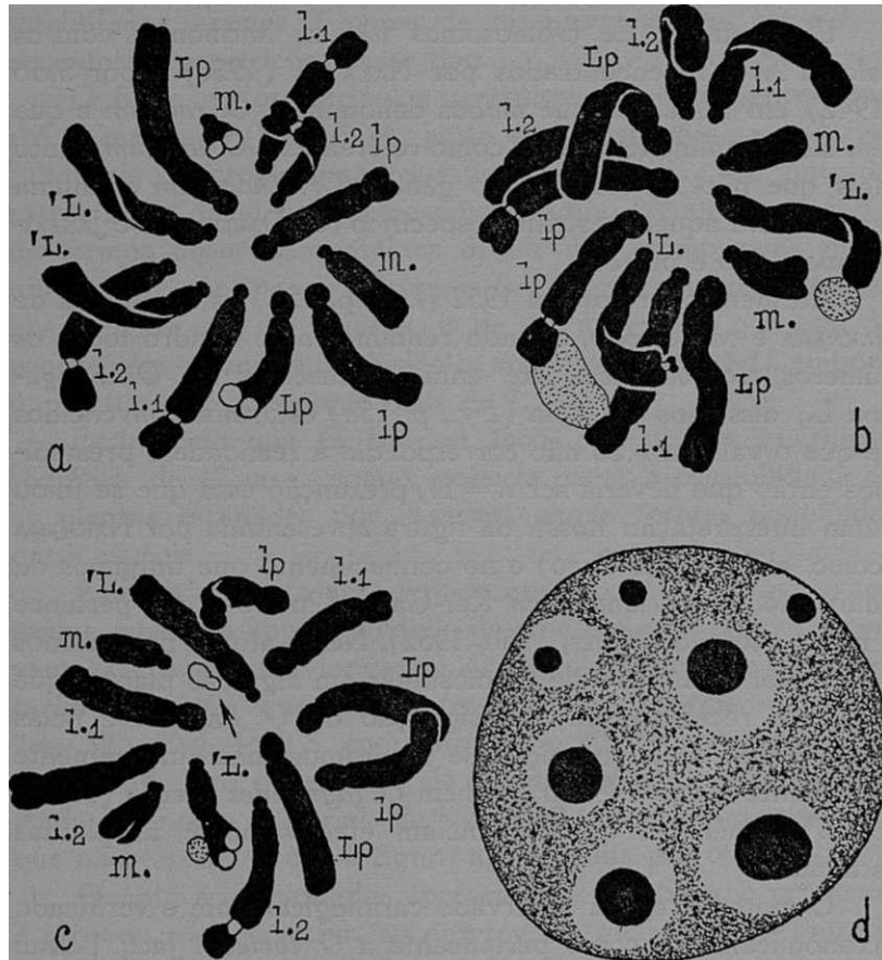
Fig. 1 — a, O. lacteum Jacq.; b, c, O. conicum Jacq. Metáfases em células dos vértices vegetativos da raiz. d, Núcleo em intercinese mostrando 7 nucléolos. Note-se em c a presença de um fragmento e em b e c a presença de nucléolos persistentes. Navachine-violete de genciana. X 3600.
