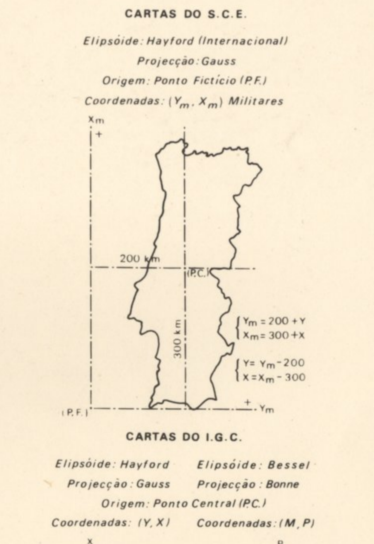
SISTEMAS DE COORDENADAS RECTANGULARES
