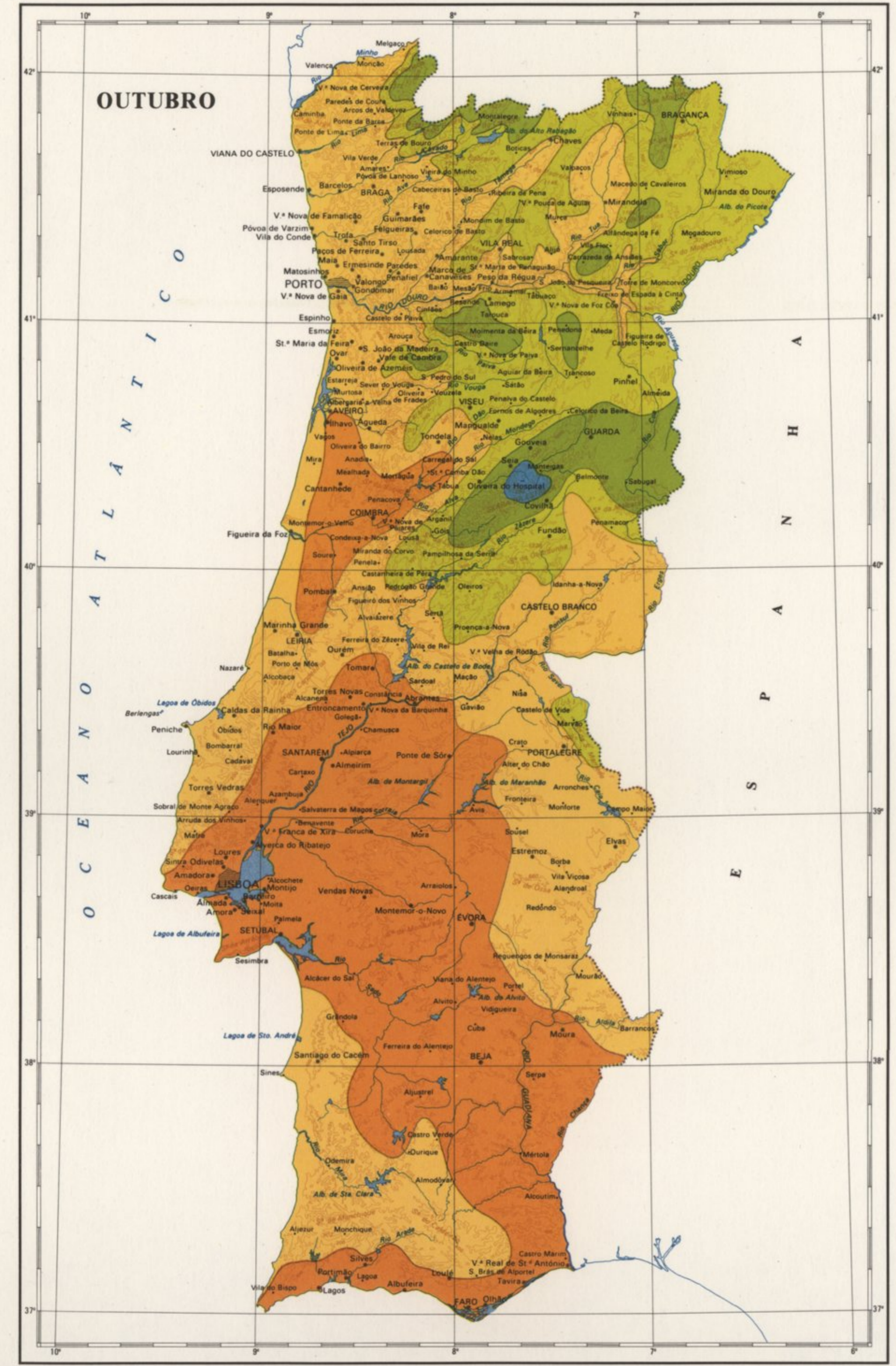
ESCALA DE SENSÇÃO BIOCLIMÁTICA (Método de Brazor/Gregorzuk)
