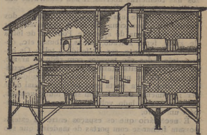
Modelo de gaiolas para reprodutoras
